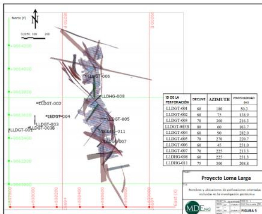
Figura 6-53 Ubicación y Orientación de las Perforaciones Geotécnicas
