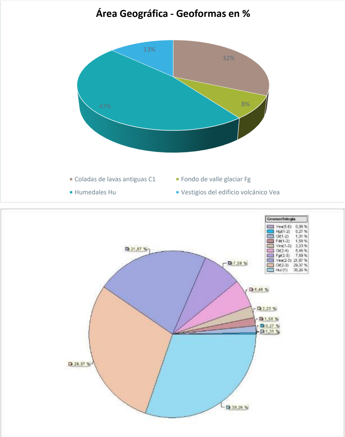
Figura 6-69 Porcentaje de las Geoformas presentes en el Área Geográfica
