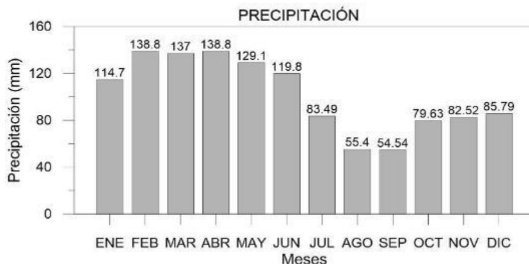
Figura 6-8 Histograma de Precipitación Mensual Estación PLL003 (2006-2019)
