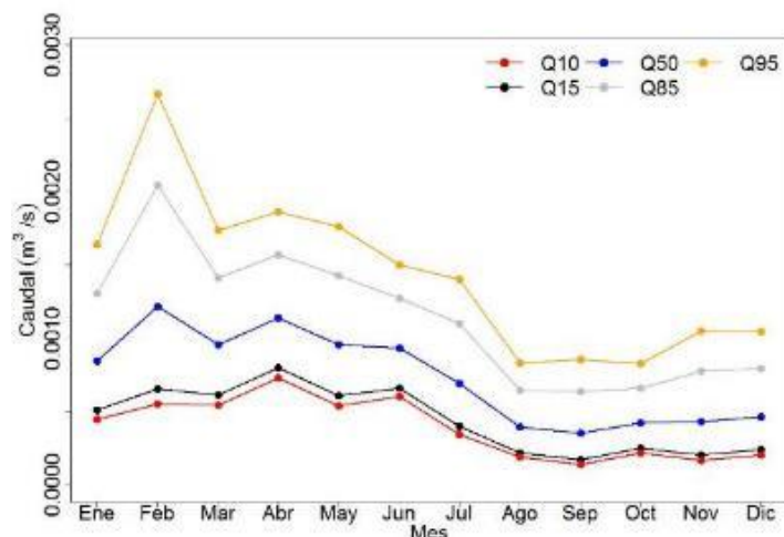
Figura 6-135 Curva de Estacionalidad correspondiente a la estación B1 para los caudales de no excedencia del 10 %, 15 %, 50 %, 85 %, y 95 %
