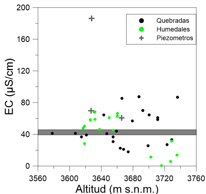
Figura 6-188 Comparación de los valores de conductividad medidos en los sitios de monitoreo y la altitud. La barra gris indica el umbral encontrado entre 44 y 46 \mu\text{S/cm} , una anomalía en valores de EC se identifica por encima del umbral y que permite identificar mananciales y zona seep.
