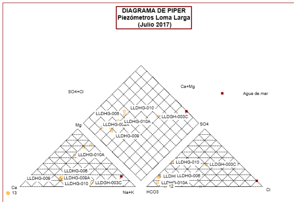
Figura 6-200 Diagrama de Piper de las Aguas Subterráneas Muestreadas en los Seis Piezómetros de Monitoreo
