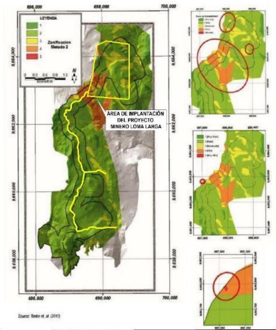
Figura 6-82 Zonas de Susceptibilidad a Deslizamientos de Tierra
