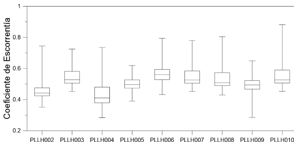
Figura 6-156 Gráfico de Cajas de los Coeficientes de Escorrentía Anuales de las Estaciones de Monitoreo Ubicadas Dentro del PLL
