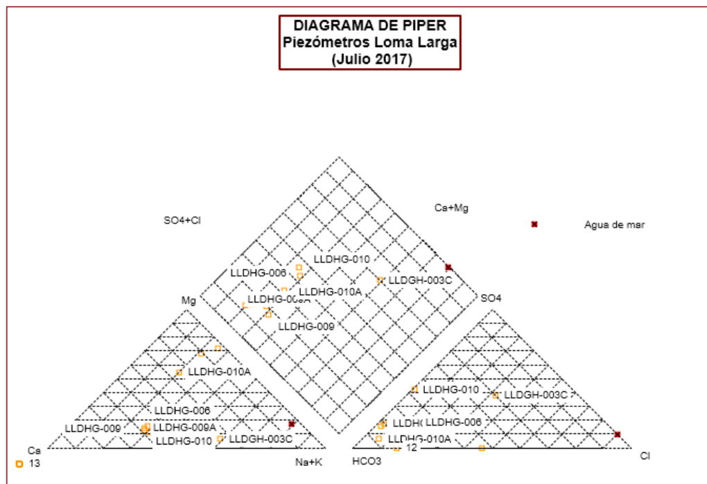
Figura 6-198 Diagrama de Piper de las Aguas Subterráneas Muestreadas en los Seis Piezómetros de Monitoreo
