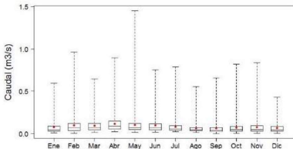
Figura 6-105 Gráfico de Cajas del Caudal Promedio Diario de Cada Mes de la Estación de Monitoreo PLLH008 durante el Periodo 1964-2020
