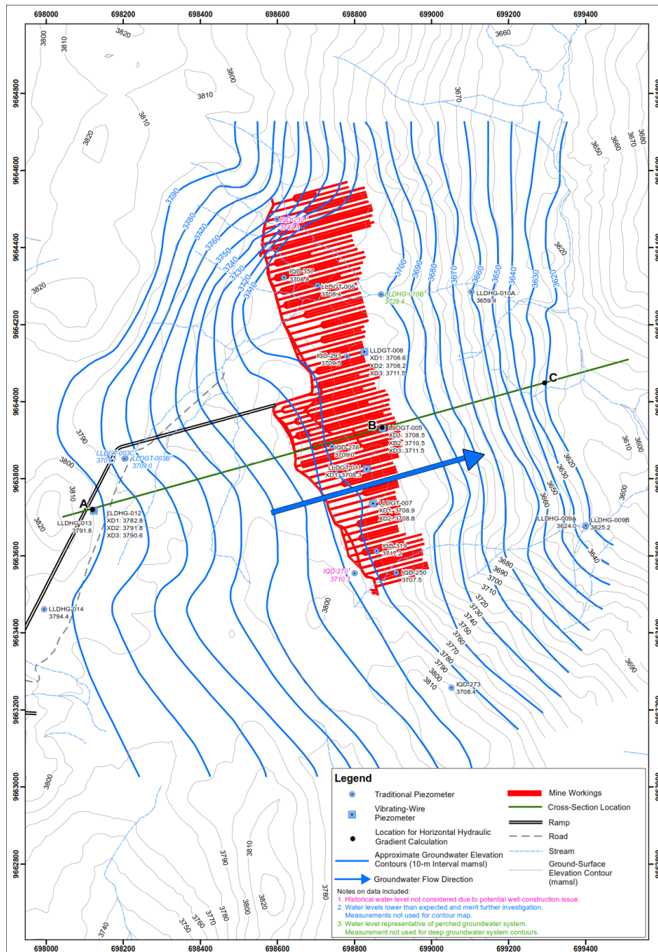
Figura 6-184 Mapa de niveles piezométricos del PLL
