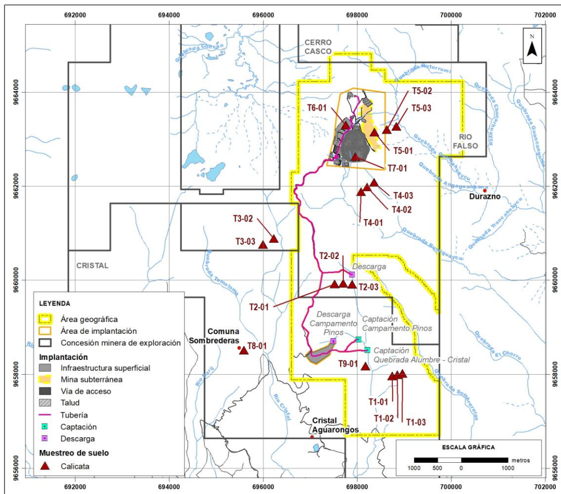
Figura 6-85 Diseño de Muestreo para la Descripción de Perfiles de Suelos en el Proyecto Loma Larga con Fines de Clasificación de Suelos
