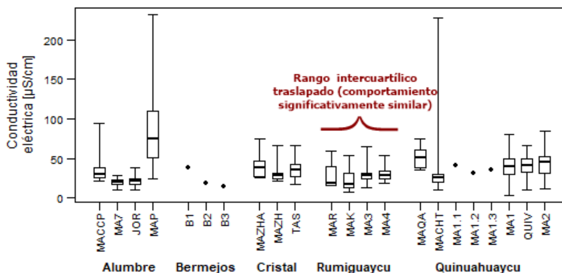
Figura 6-166 Agrupación de Puntos de Muestreo por Rango Intercuartílico
