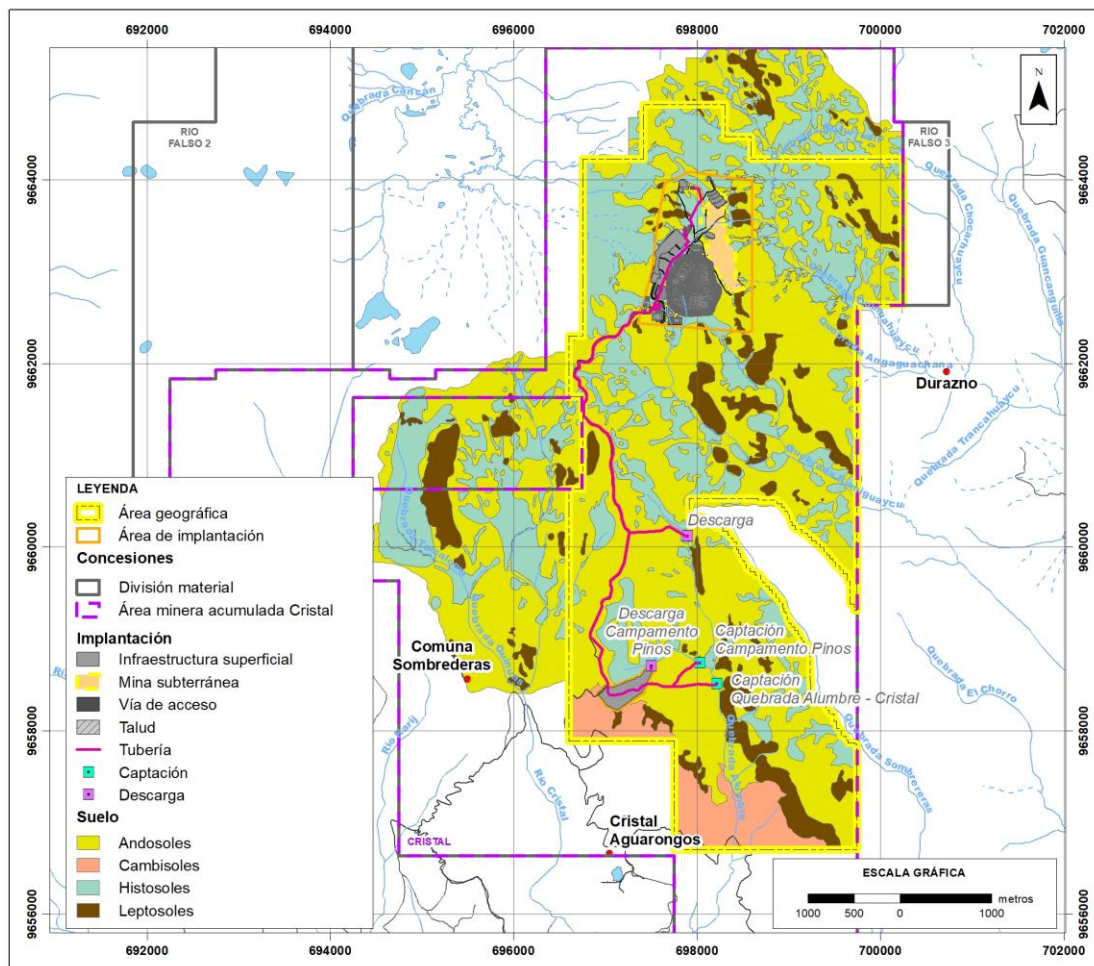
Figura 6-89 Mapa de Suelos según la Base Referencial Mundial del Recurso Suelo para el Proyecto Loma Larga
