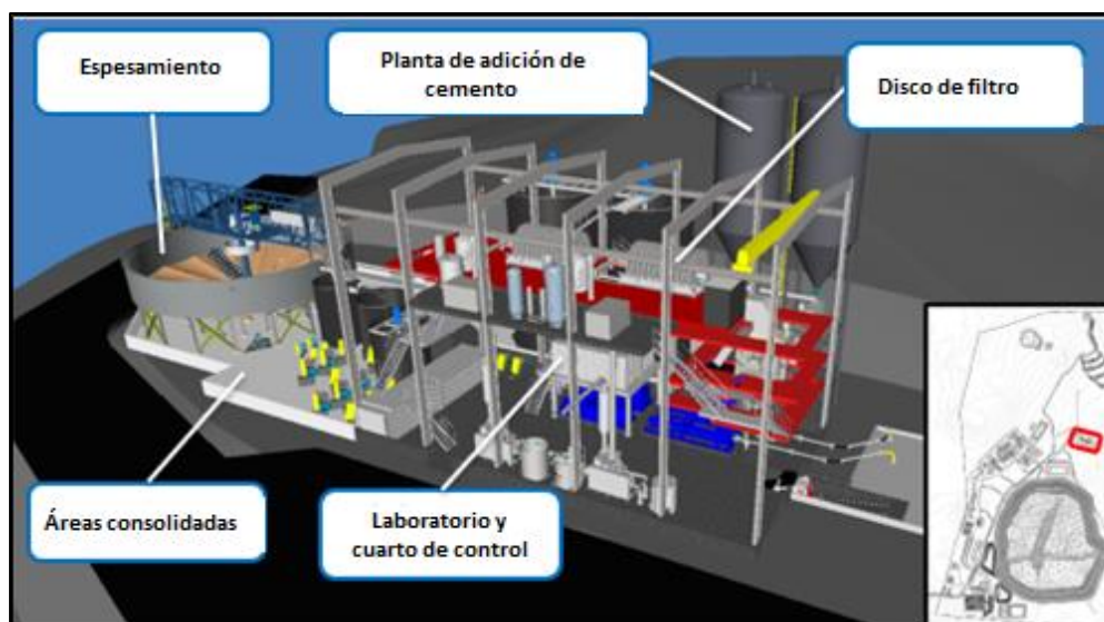
Figura 7-66 Diseño de la Planta de Relleno en Pasta
