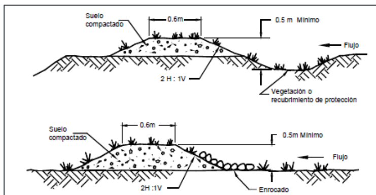
Figura 7-87 Bermas de Desvío Típicas
