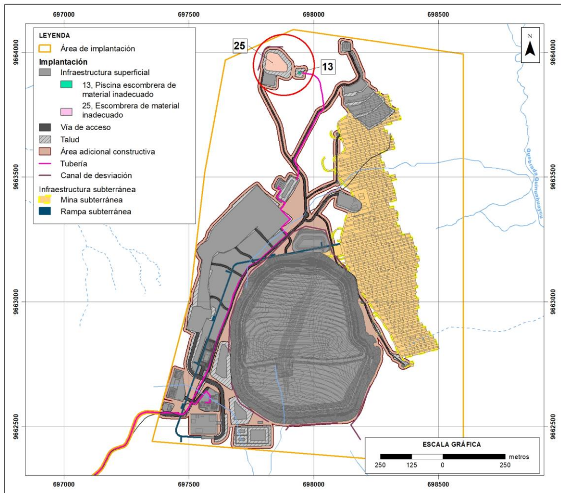
Figura 7-112 Ubicación de la Escombrera de Material Inadecuado
