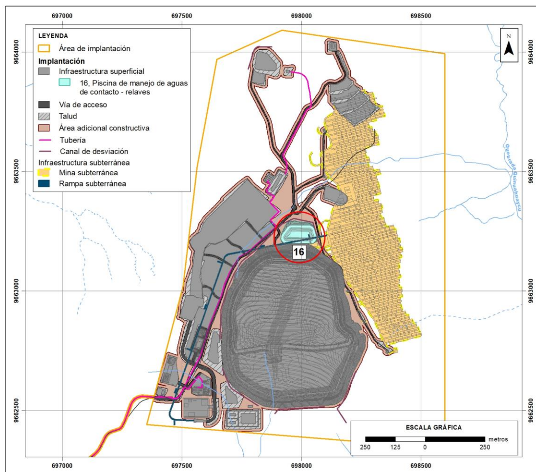
Figura 7-103 Ubicación de la Piscina de Manejo de Aguas de Contacto con Relaves
