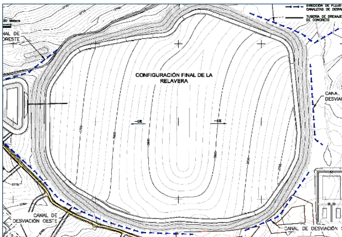
Figura 7-115 Cierre de la Relavera-Configuración Final
