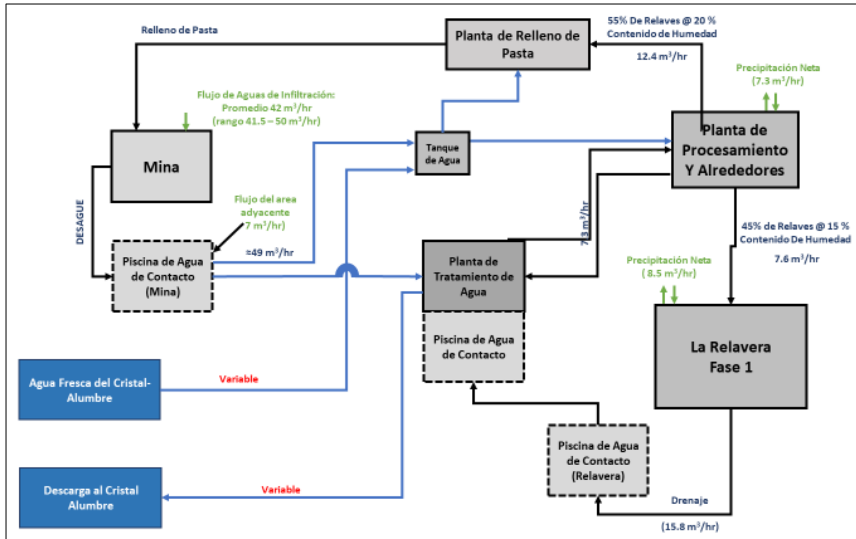
Figura 7-98 Diagrama de Flujo Esquemático para la Etapa Operativa (Relavera Fase 1) del PLL
