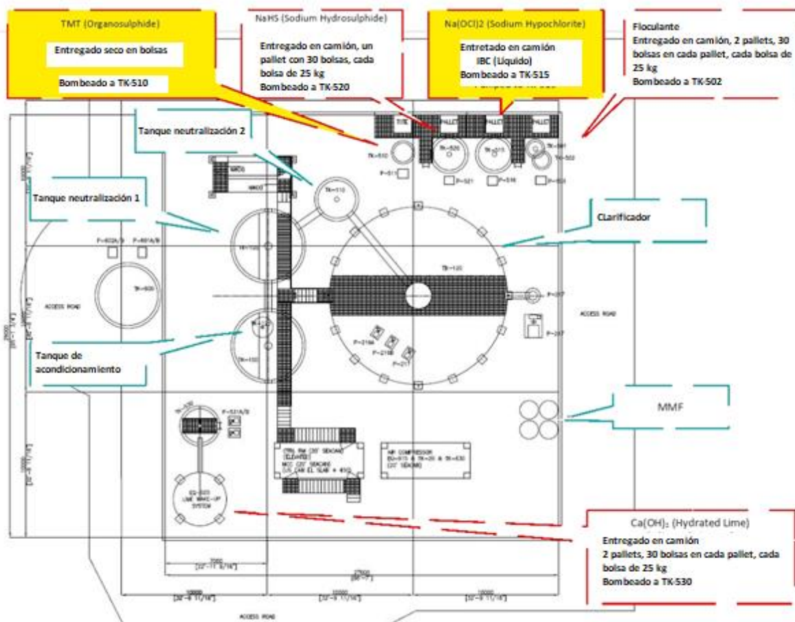
Figura 7-107 Implantación General de la PTA
