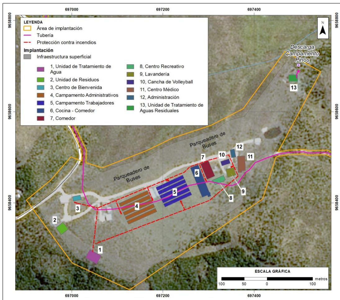
Figura 7-76 Acondicionamiento Tipo del Campamento Pinos
