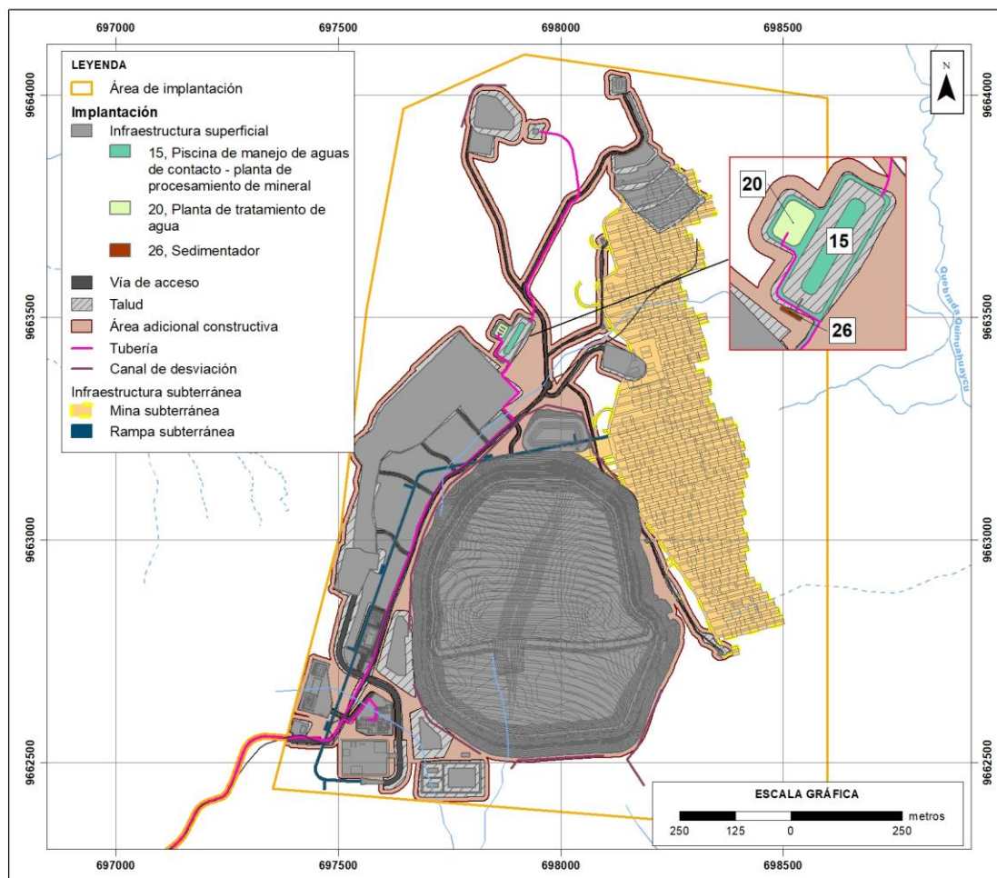
Figura 7-106 Ubicación de la Planta de Tratamiento de Agua
