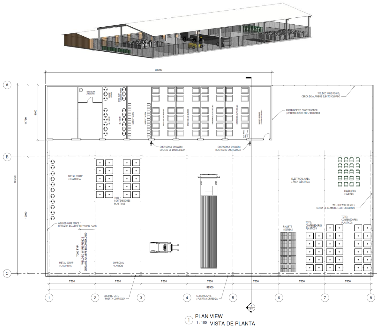
Figura 7-110 Diseño tipo del Área para almacenamiento temporal de residuos
