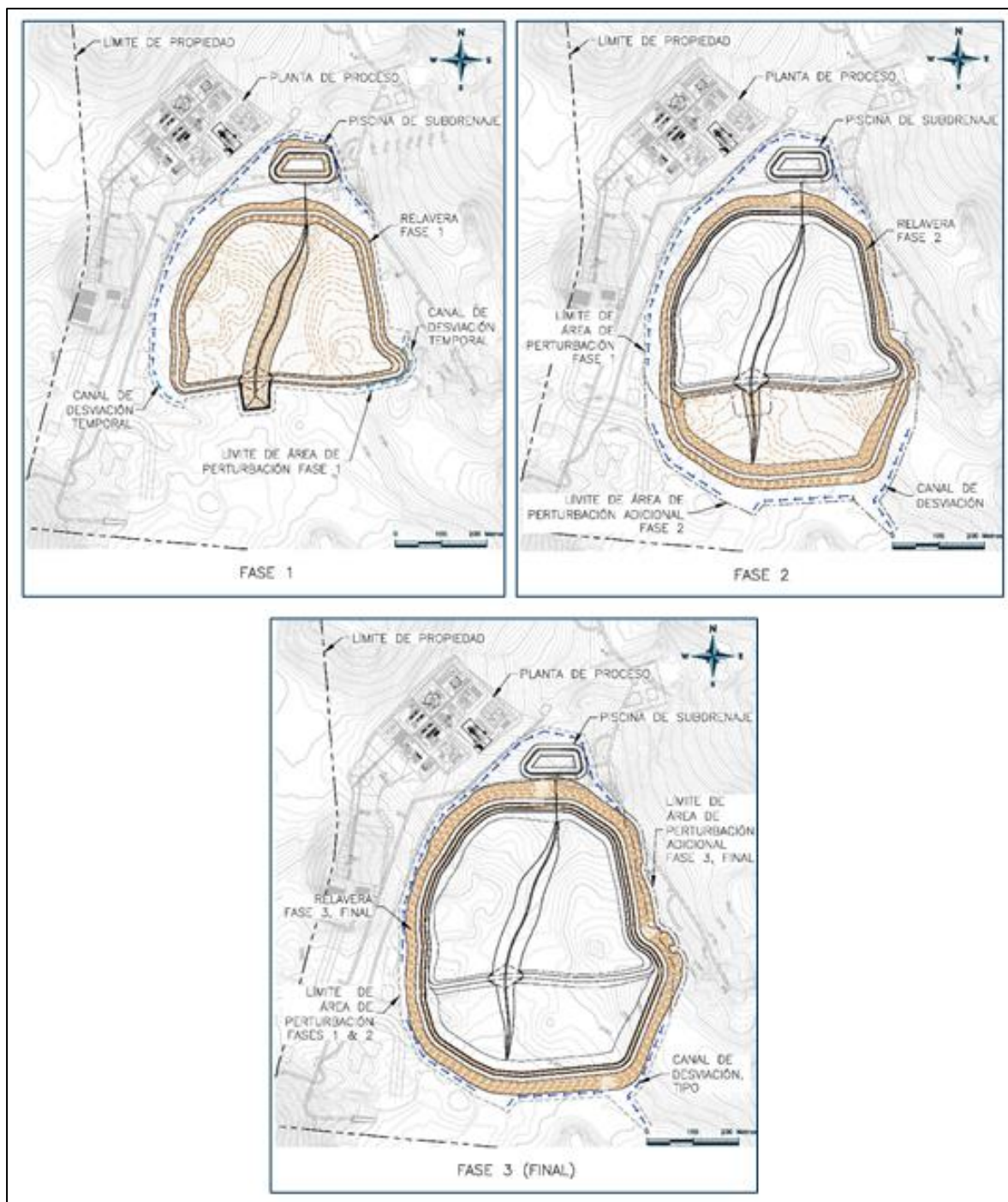
Figura 7-57 Fases de Construcción de la Relavera
