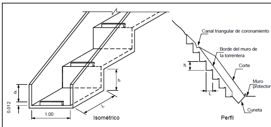
Figura 7-94 Canales en Gradería con Disipación de Energía
