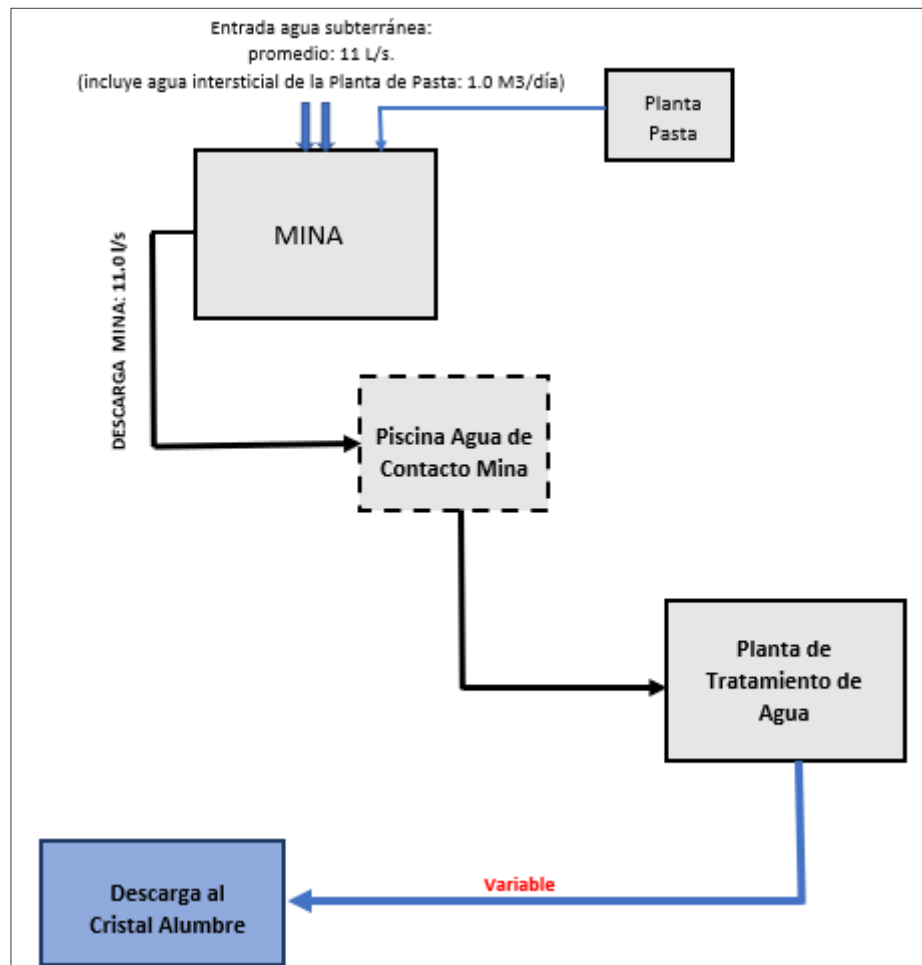
Figura 7-101 Diagrama de Flujo Esquemático Balance de Agua para el Área de la Mina y Áreas Adyacentes del PLL
