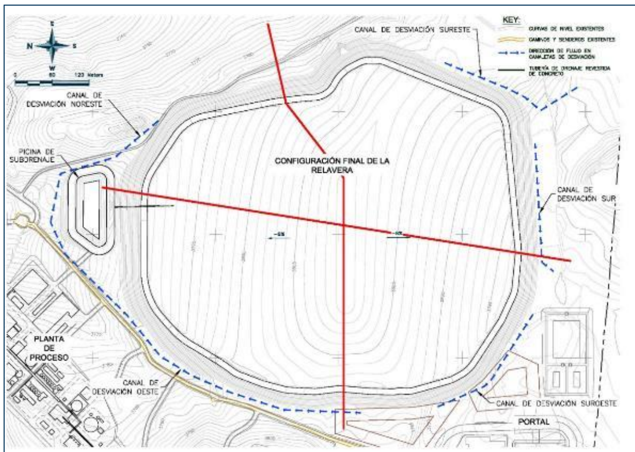
Figura 7-60 Ubicación de Secciones para el Análisis de Estabilidad
