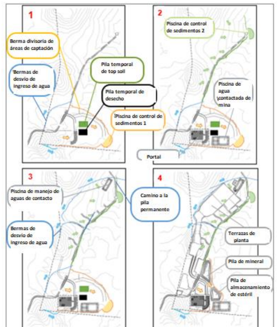
Figura 7-114 Secuencia de Construcción de la Mina y de la Planta de Procesamiento de Mineral
