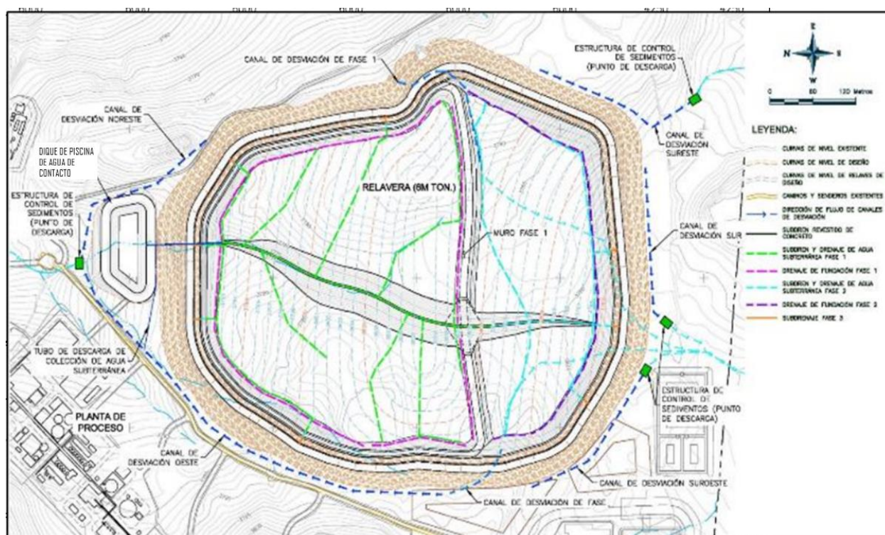
Figura 7-56 Planta General de la Relavera
