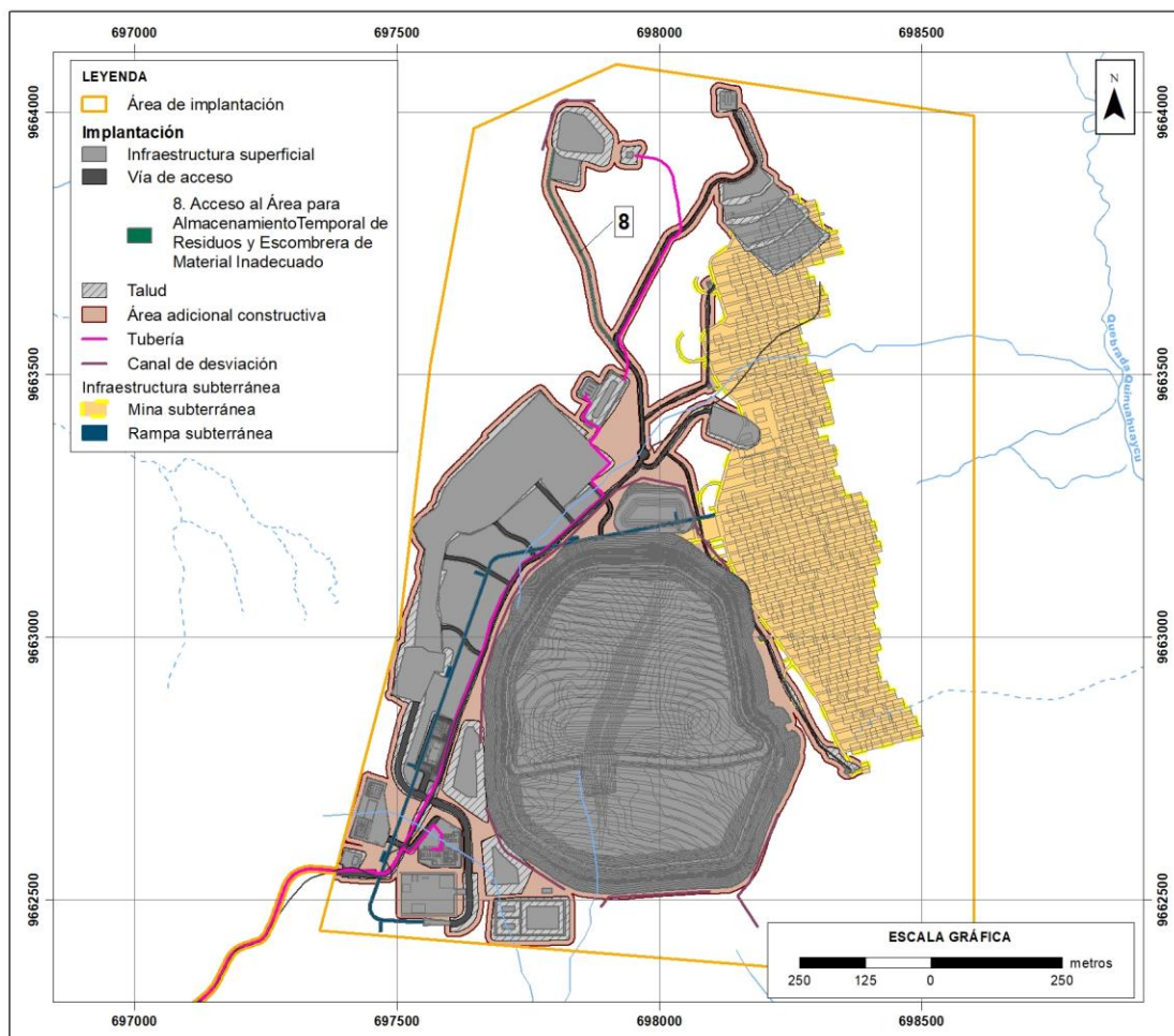
Figura 7-74 Ubicación del Acceso al Área para Almacenamiento Temporal de Residuos y Escombrera de Material Inadecuado
