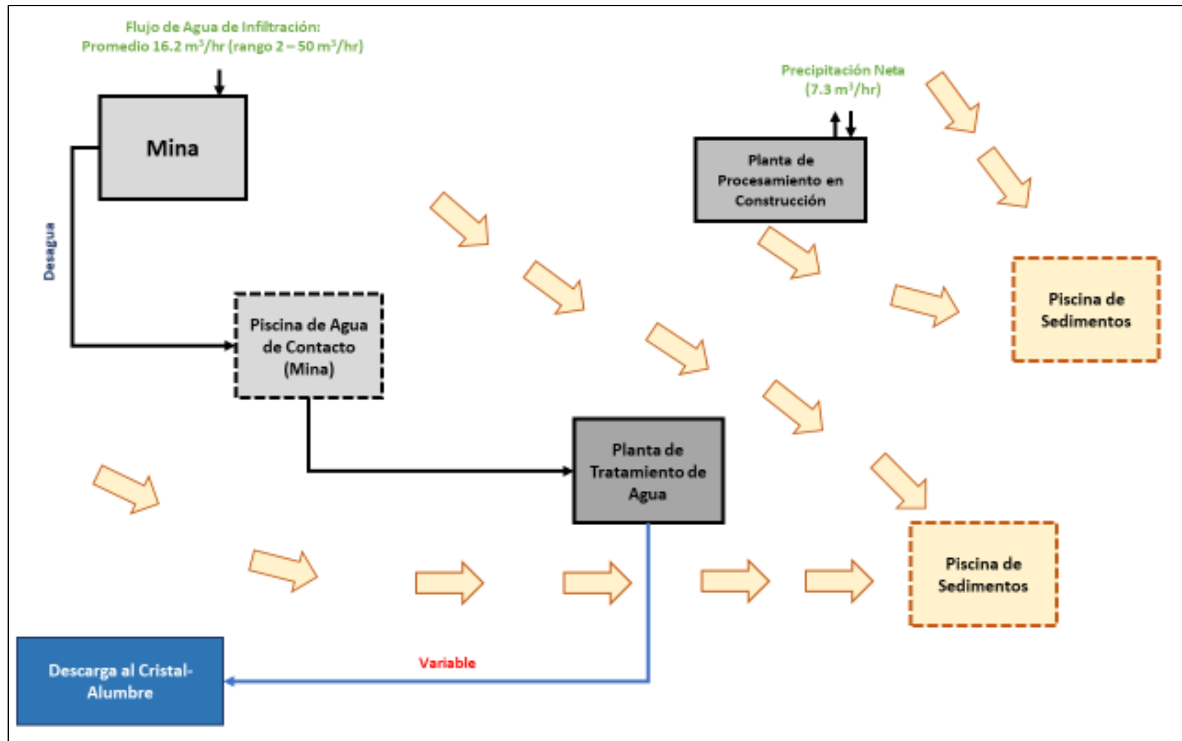
Figura 7-97 Diagrama de Flujo Esquemático para la Etapa de Construcción del PLL
