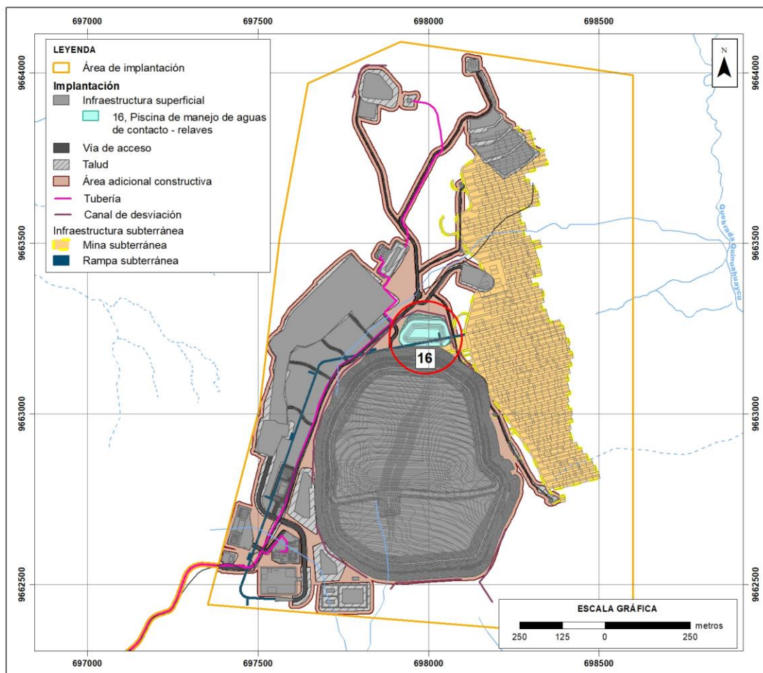
Figura 7-63 Ubicación de la Piscina de Agua de Contacto de la Relavera
