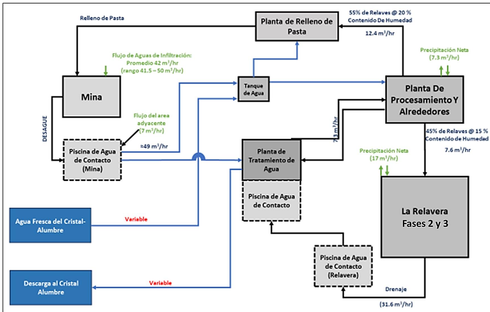
Figura 7-99 Diagrama de Flujo Esquemático para la Etapa Operativa (Relavera Fases 2 y 3) del PLL
