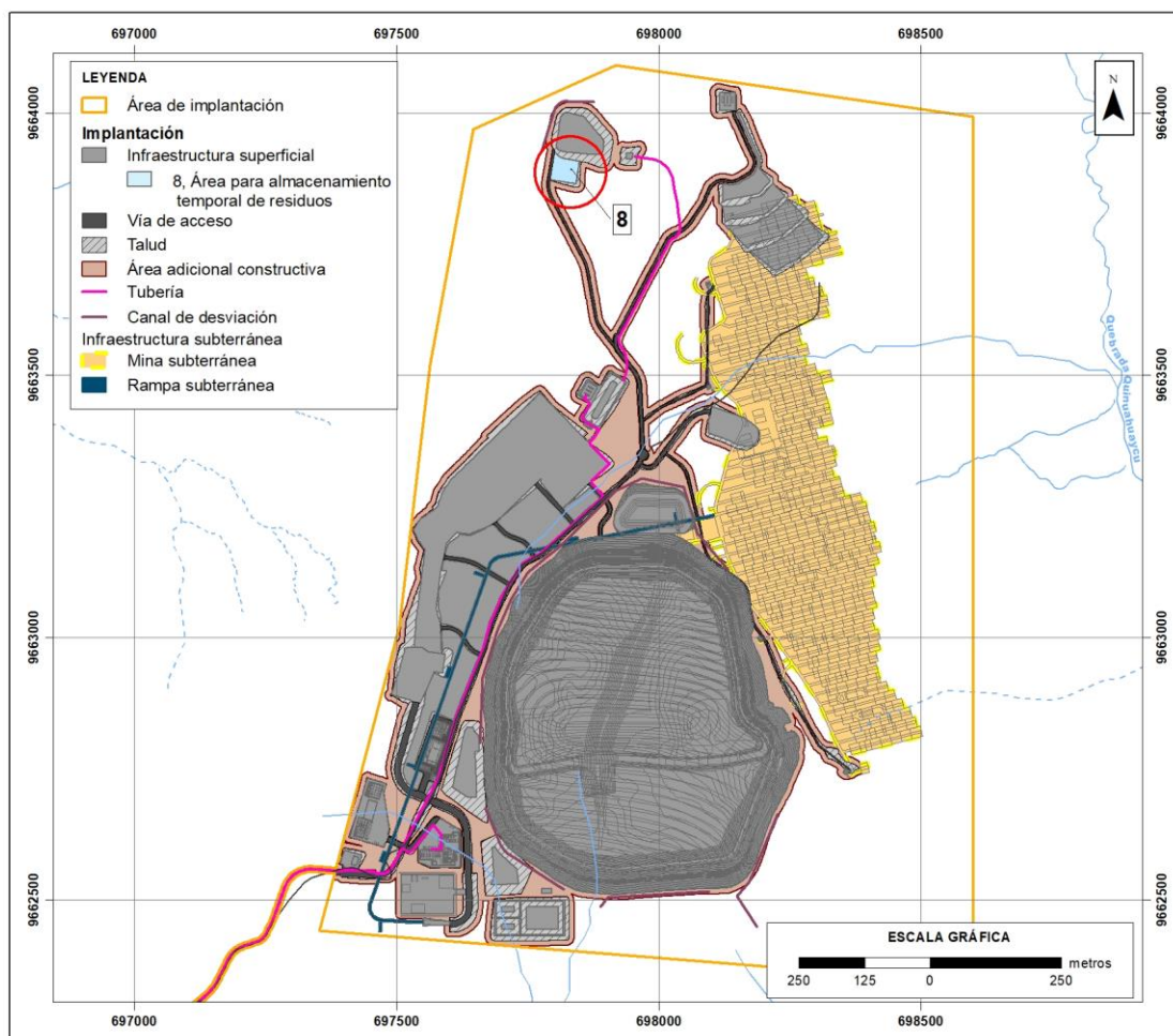
Figura 7-109 Ubicación del Área para Almacenamiento Temporal de Residuos
