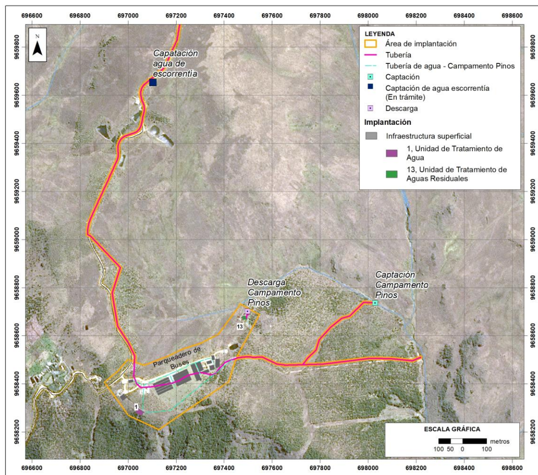
Figura 7-77 Ubicación de los Puntos de Captación y Descarga de Agua del Campamento Pinos
