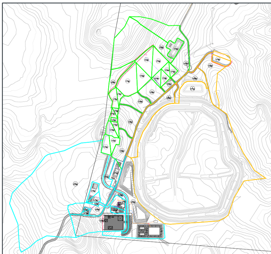
Figura 7-86 Ubicación de Obras Superficiales de Drenaje
