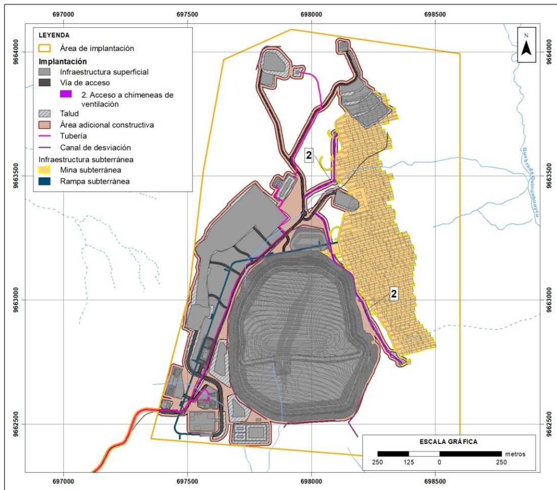
Figura 7-71 Ubicación del Acceso a las Chimeneas
