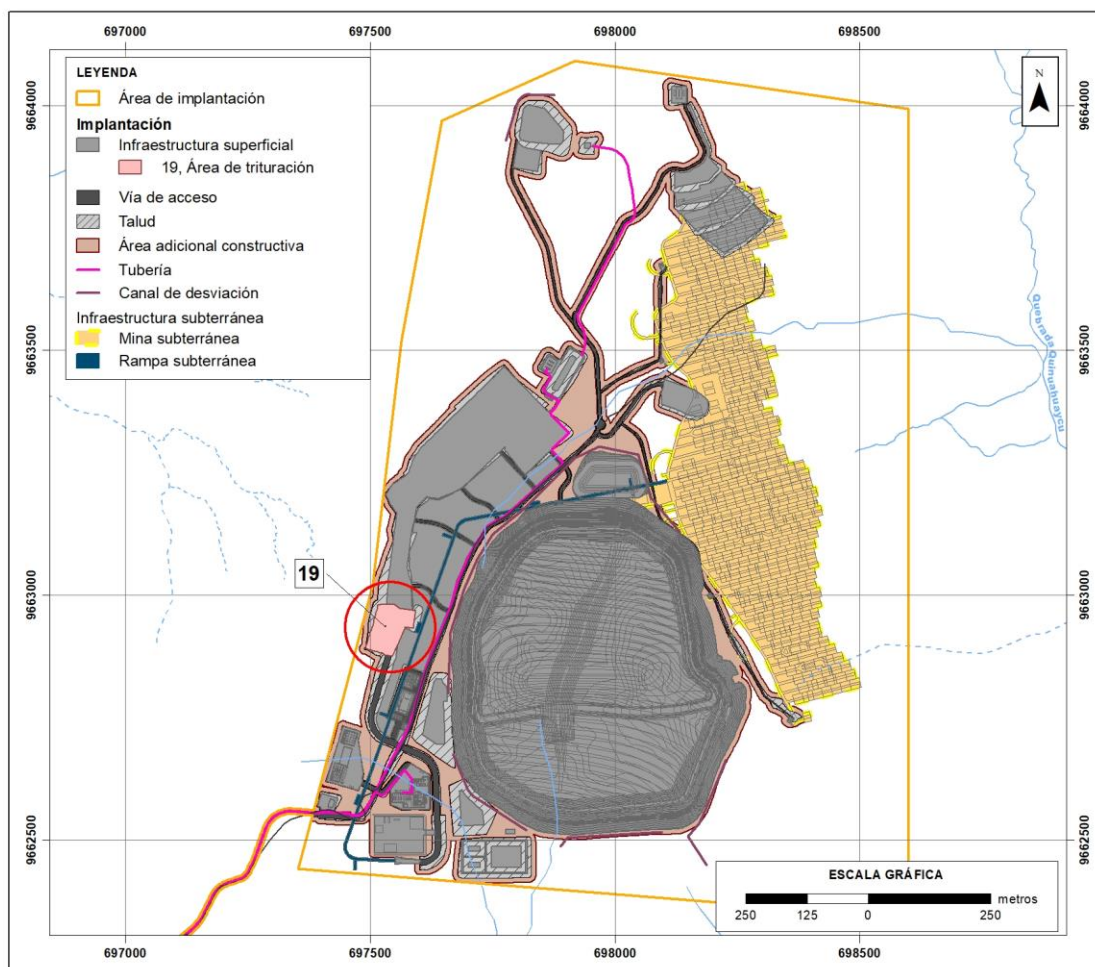
Figura 7-36 Ubicación del Área de Trituración
