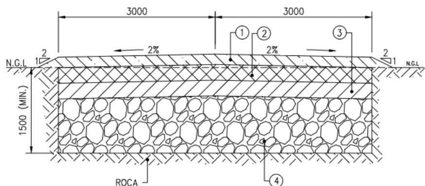
Figura 7-54 Diseño típico para la construcción de las rutas internas
