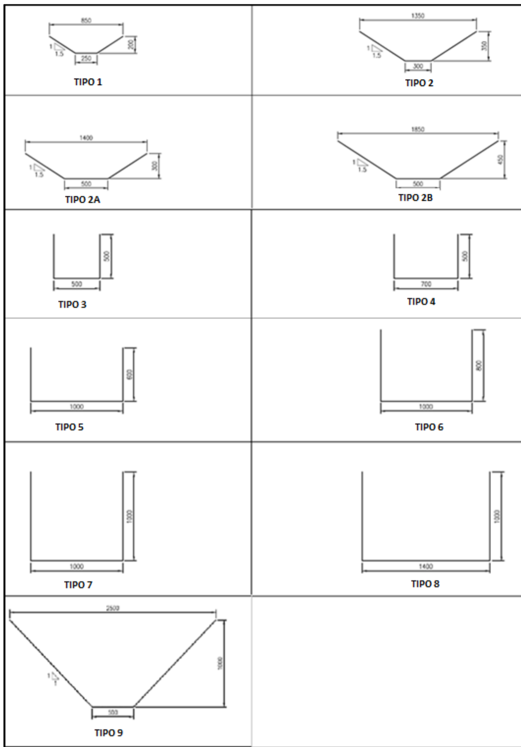
Figura 7-91 Cunetas y Canales Tipo
