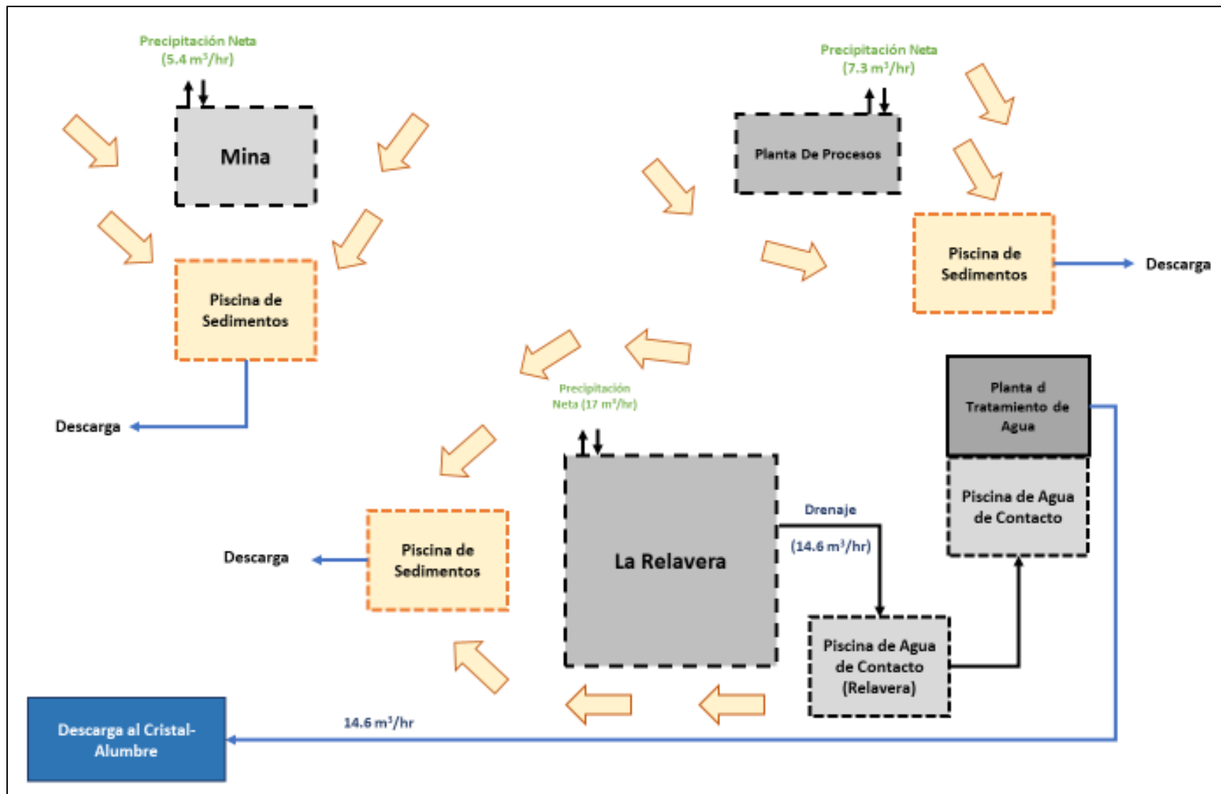
Figura 7-100 Diagrama de Flujo Esquemático para la Etapa de Cierre del PLL
