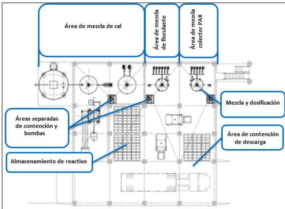
Figura 7-75 Diseño del Edificio de Reactivo Seco y del Edificio del Reactivo Líquido
