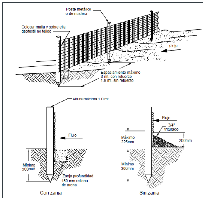
Figura 7-89 Barrera Perimetral con Filtro Típica
