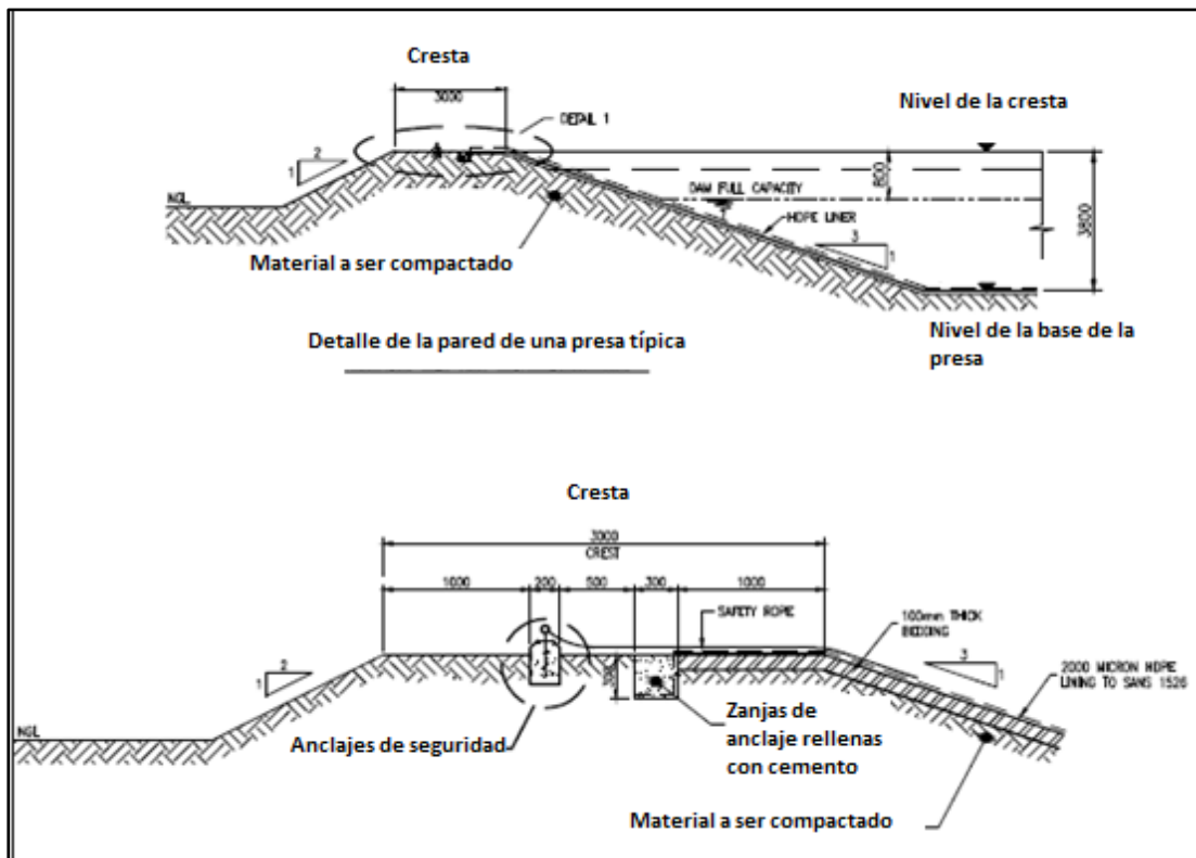
Figura 7-95 Piscinas Típicas para el Proyecto
