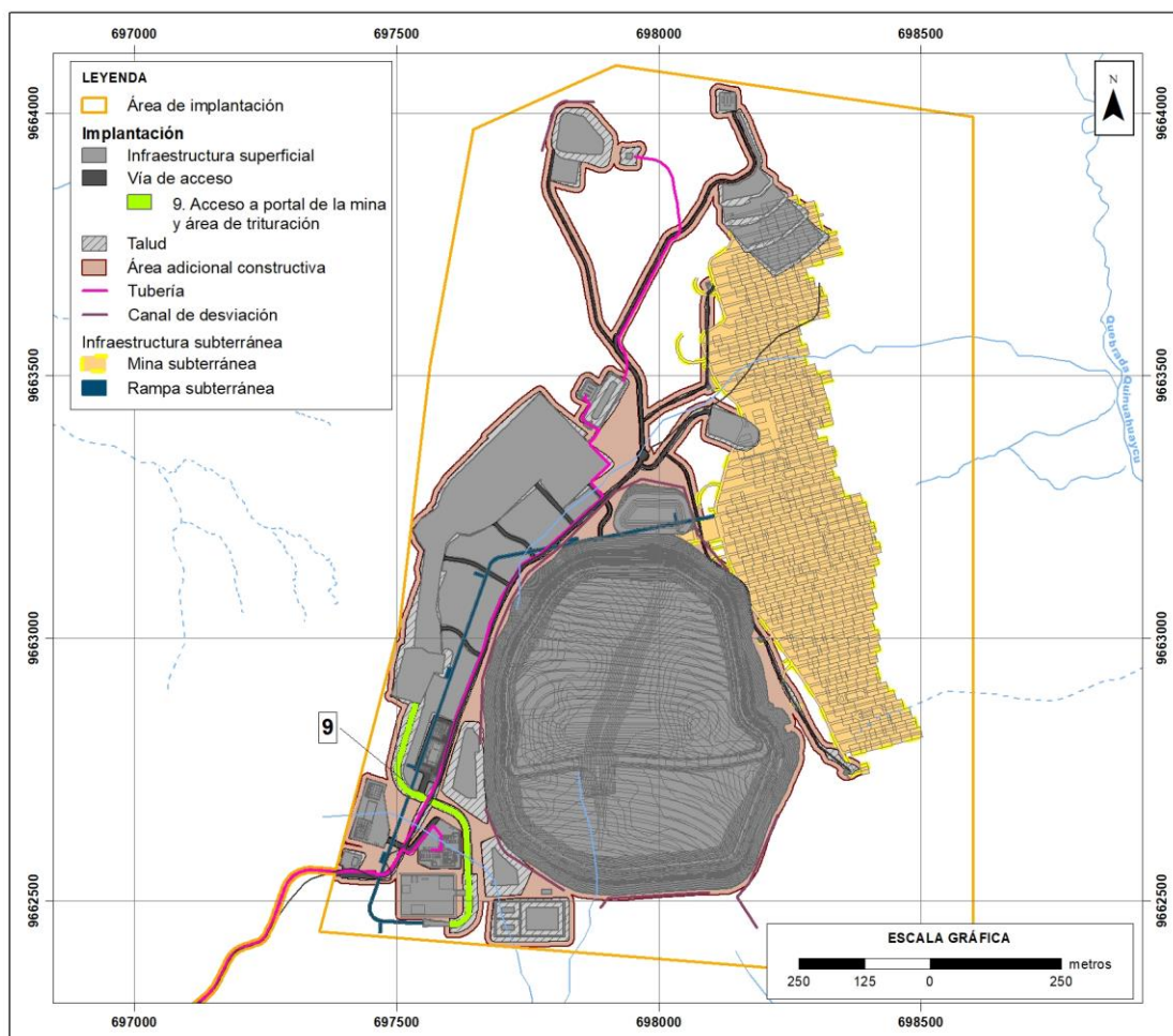
Figura 7-69 Ubicación del Acceso al Portal de la Mina y Área de Trituración
