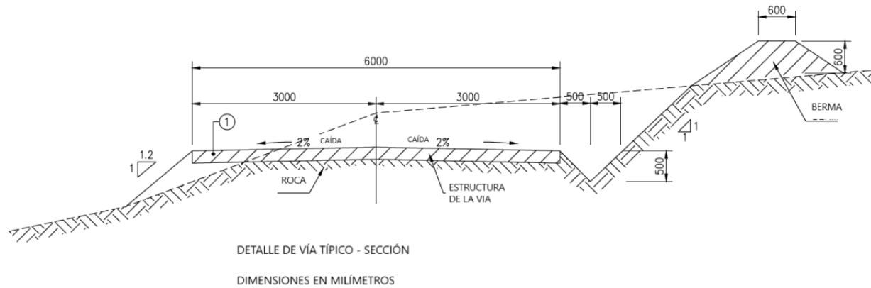
Figura 7-67 Criterio de diseño de las vías internas
