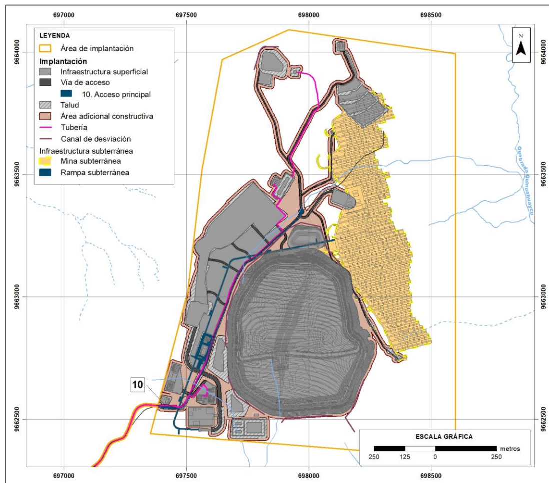
Figura 7-68 Ubicación del Acceso Principal
