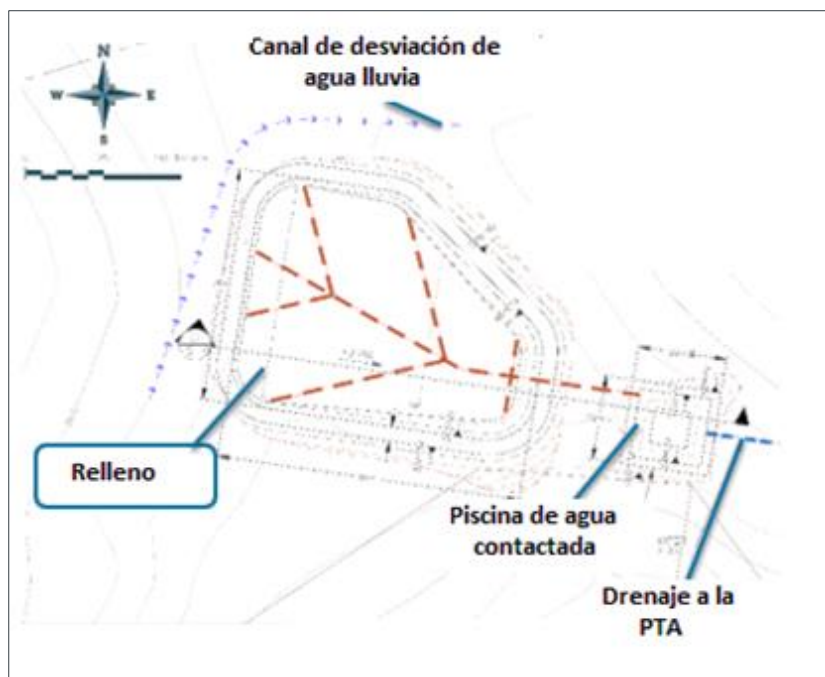
Figura 7-113 Zonas de Manejo de Escorrentía-Captación y Desvío de Agua en el Sitio
