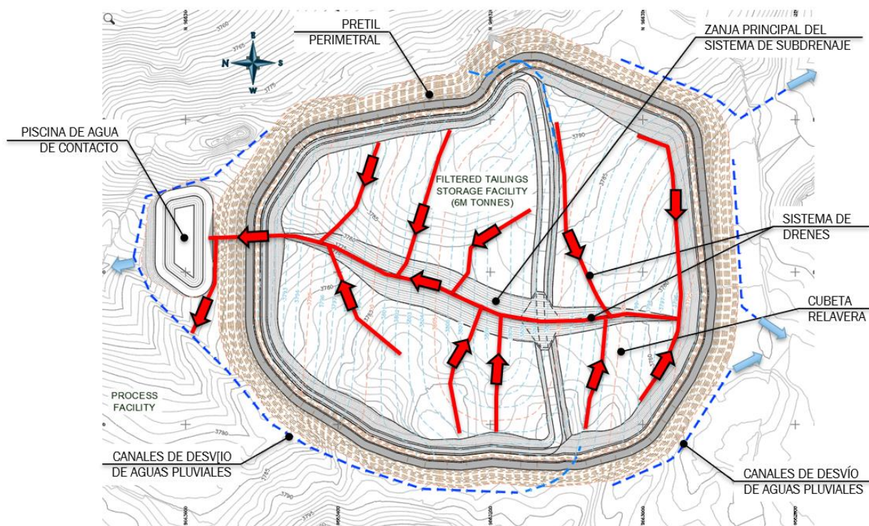
Figura 7-61 Planta del sistema de manejo de aguas subterráneas
