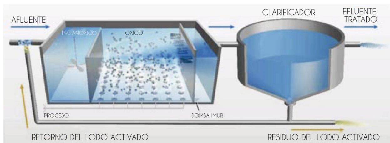
Figura 7-105 Esquema de Sistema de Tratamiento de Aguas Residuales con Lodos Activados
