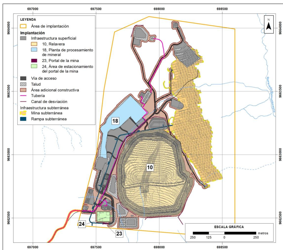
Figura 7-96 Distribución General de las Tres Áreas Principales para el Manejo de Agua del Sitio
