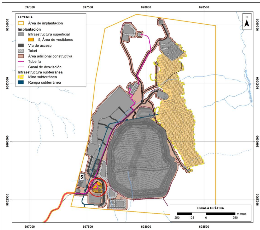
Figura 7-30 Ubicación del Área de Vestidores
