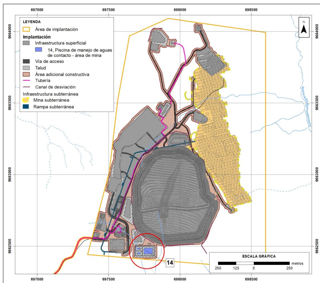
Figura 7-17 Ubicación de la Piscina de Manejo de Aguas de Contacto - Área de Mina
