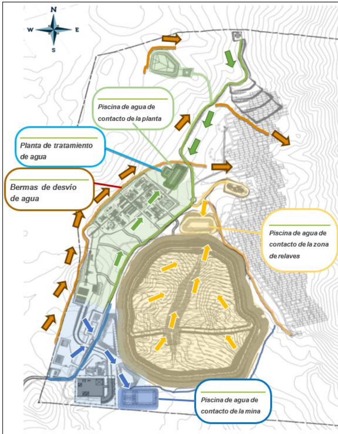
Figura 7-83 Zonas de Manejo de Escorrentía-Captación y Desvío de Agua en el Sitio
