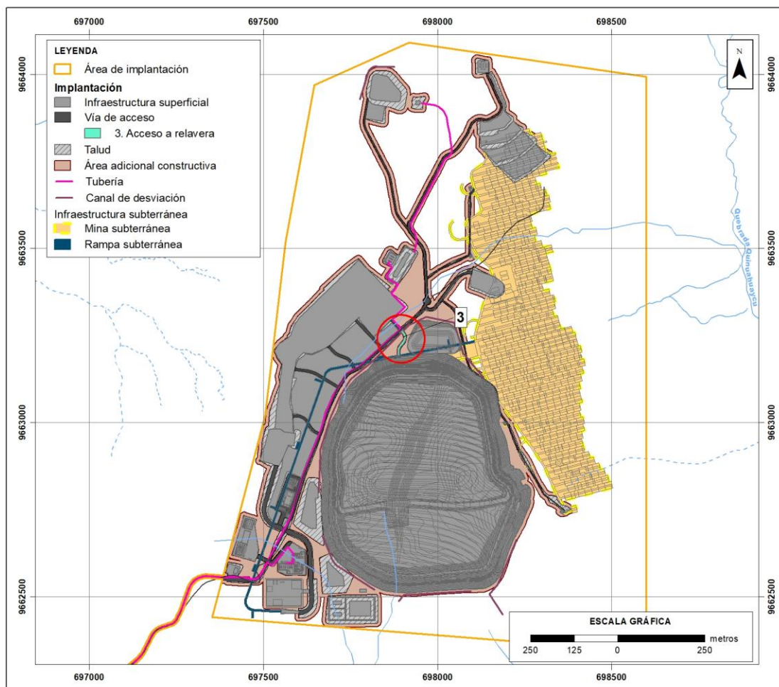
Figura 7-64 Ubicación de la Vía de Acceso a la Relavera
