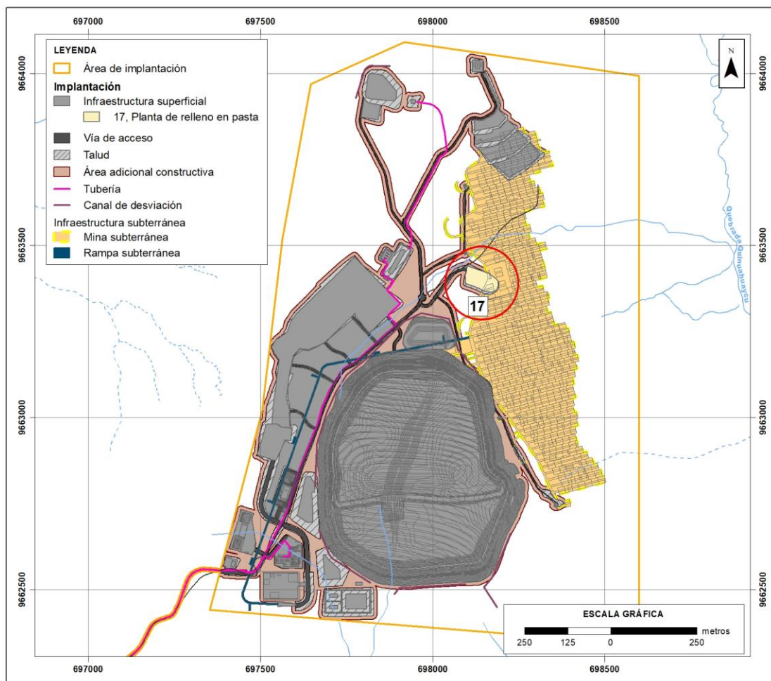
Figura 7-65 Ubicación de la Planta de Relleno en Pasta
