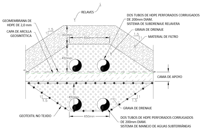
Figura 7-62 Sección típica del dren del sistema de manejo de aguas subterráneas
