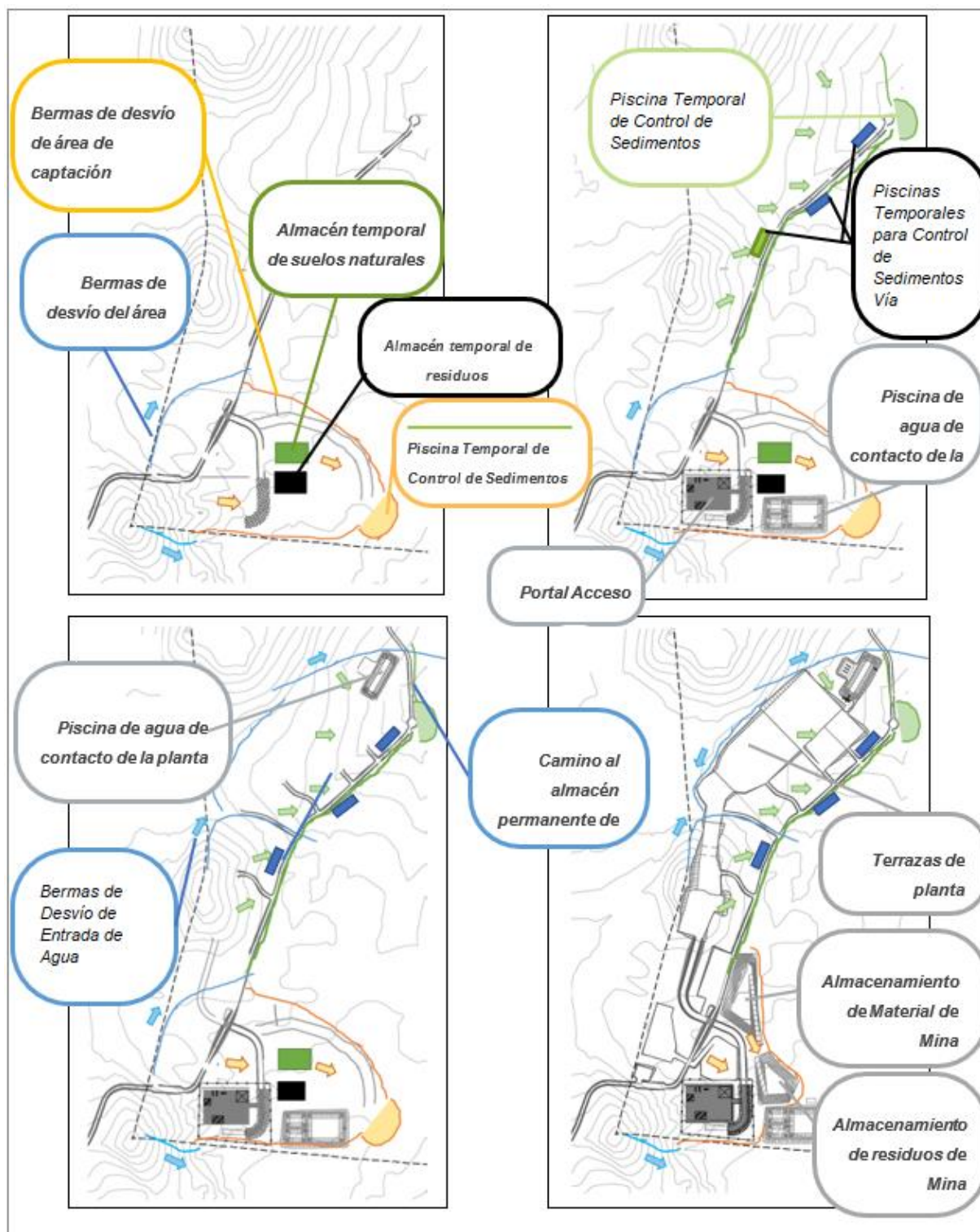
Figura 7-85 Secuencia de Construcción de la Mina y la Planta de Procesamiento de Mineral
