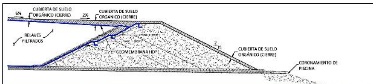
Figura 7-116 Cierre de la Relavera-Sección Muro y Piscina
