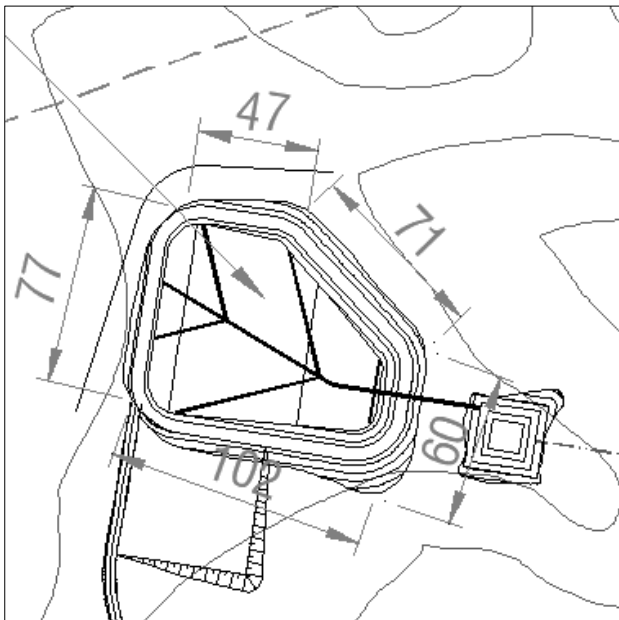
Figura 7-111 Dimensiones de la escombrera de material inadecuado y piscina de sedimentación
