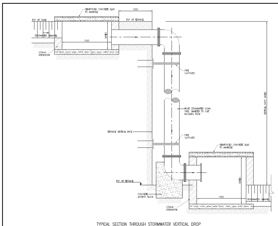
Figura 7-93 Cámaras de Caídas Verticales
