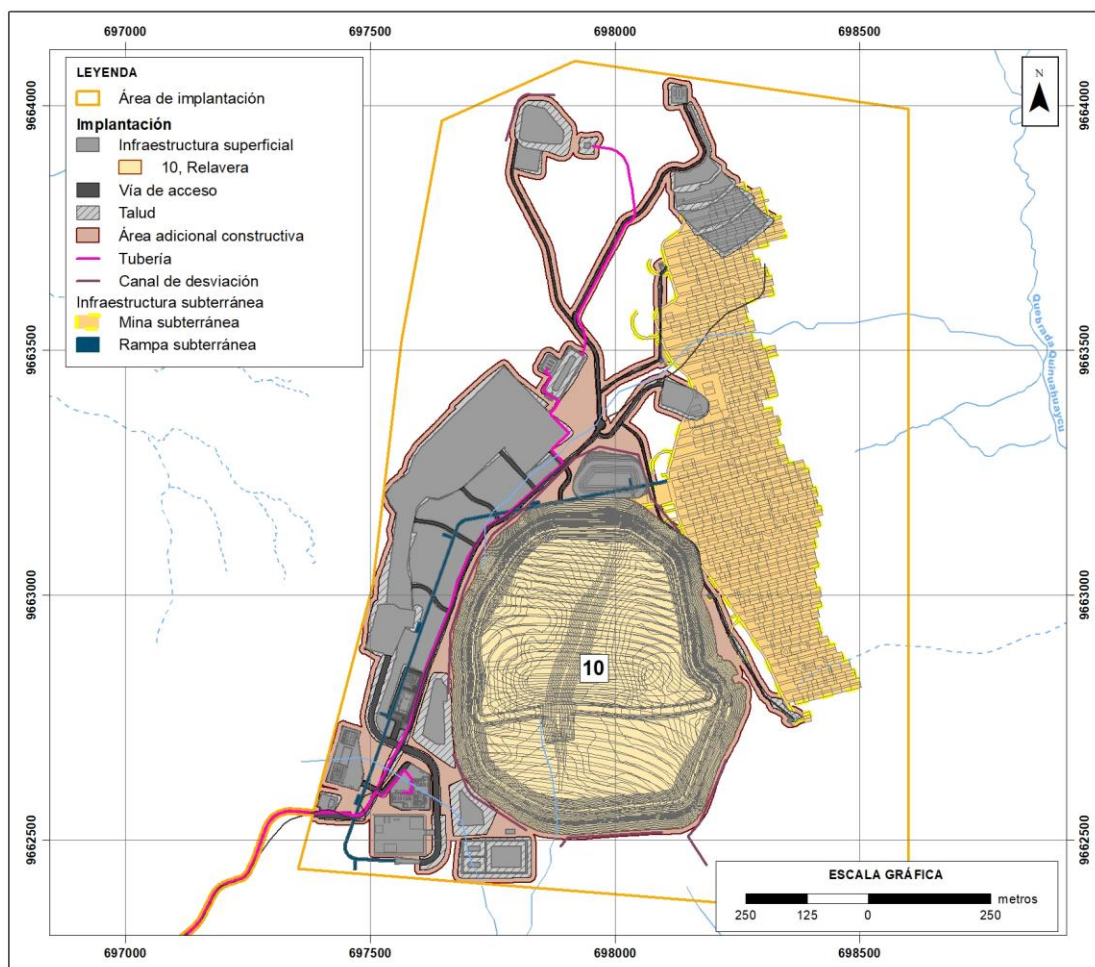
Figura 7-55 Ubicación de la Relavera
