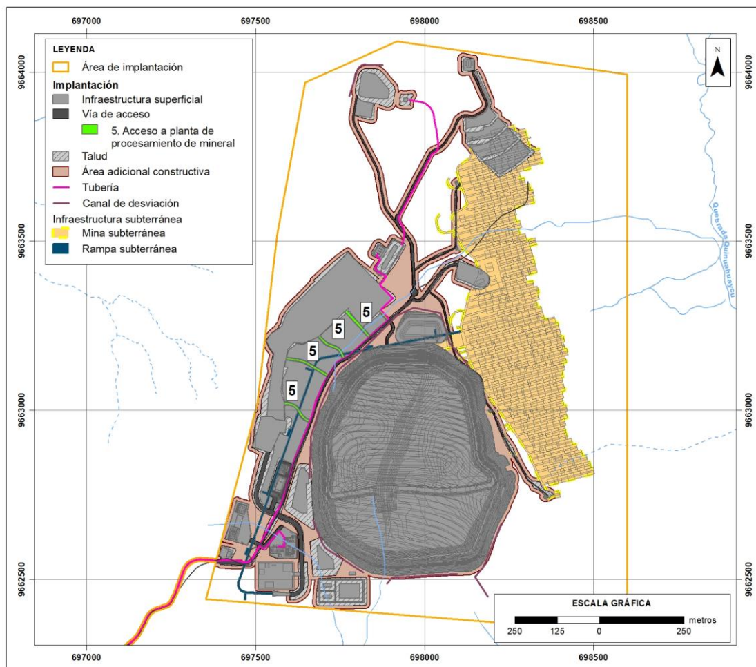
Figura 7-72 Ubicación de los Accesos a la Planta de Procesamiento de Mineral
