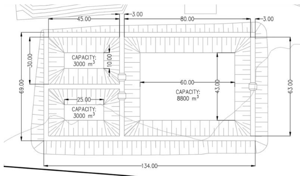
Figura 7-102 Sistema de desagüe de mina para tratamiento de aguas
