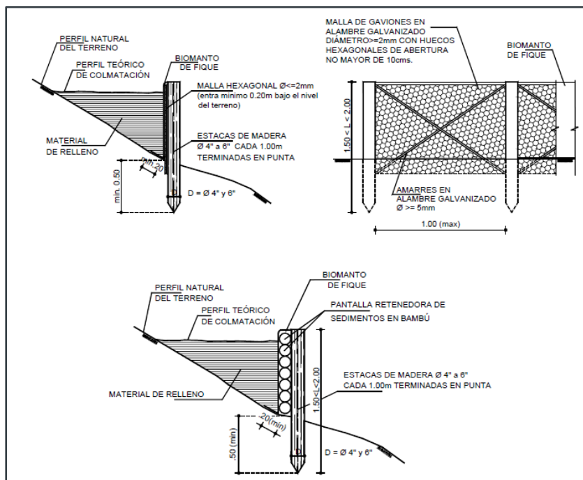
Figura 7-88 Trinchos Típicos para Restablecer Cobertura en Zonas de Alta Pendiente
